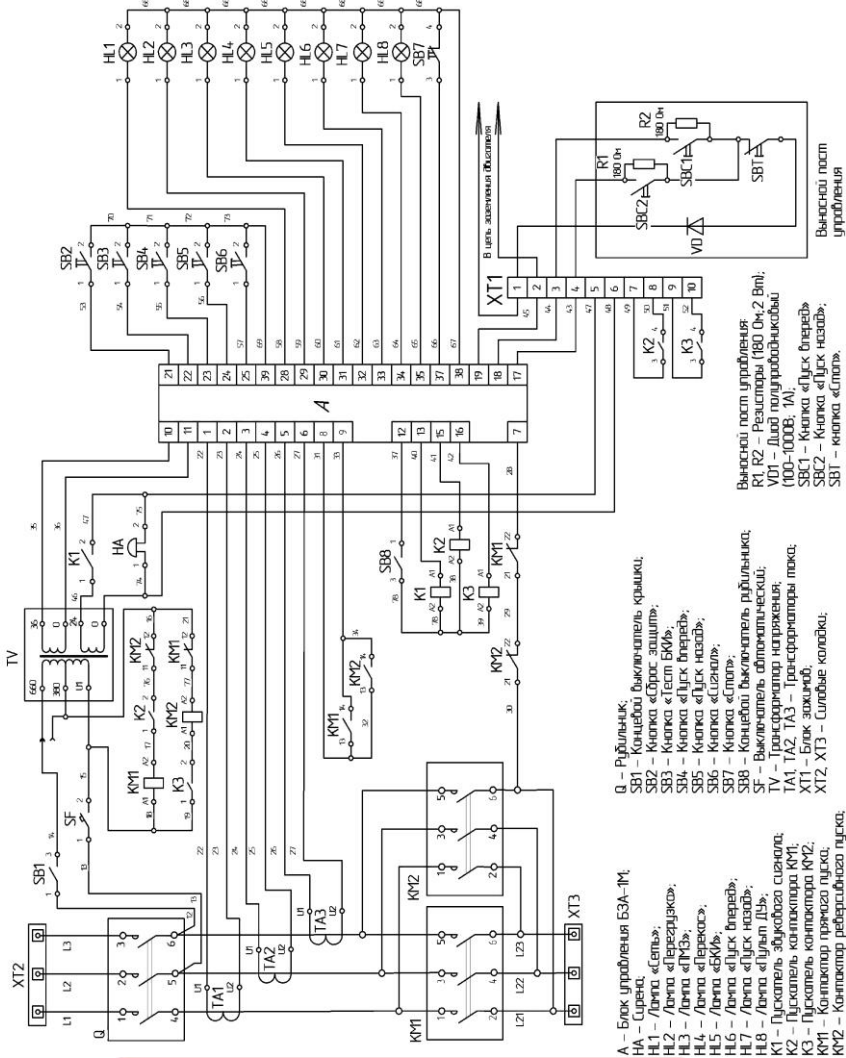
Рисунок 4. Схема ДЗРА.656439.026 ЭЗ. ПРН-Р-М
