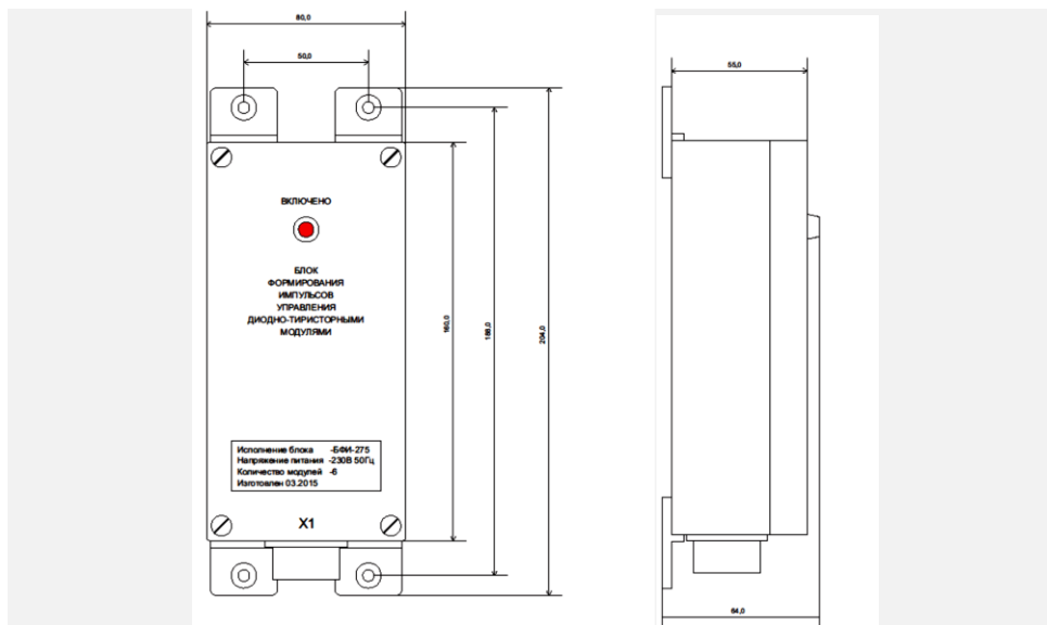
Рисунок 2. Внешний вид и габаритные размеры БФИ-275
