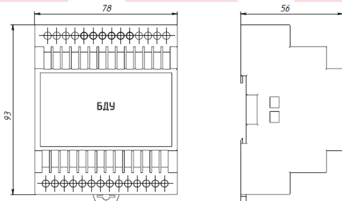
Рисунок 1. Общий вид и габаритные размеры БДУ-М
