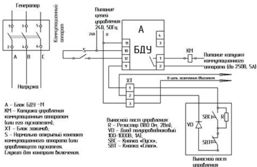
Рисунок 2. Возможный вариант схемы включения блока в НКУ
