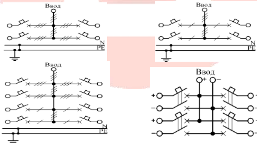
Приложение 1 Принципиальная электрическая схема ПР без выключателей ввода
