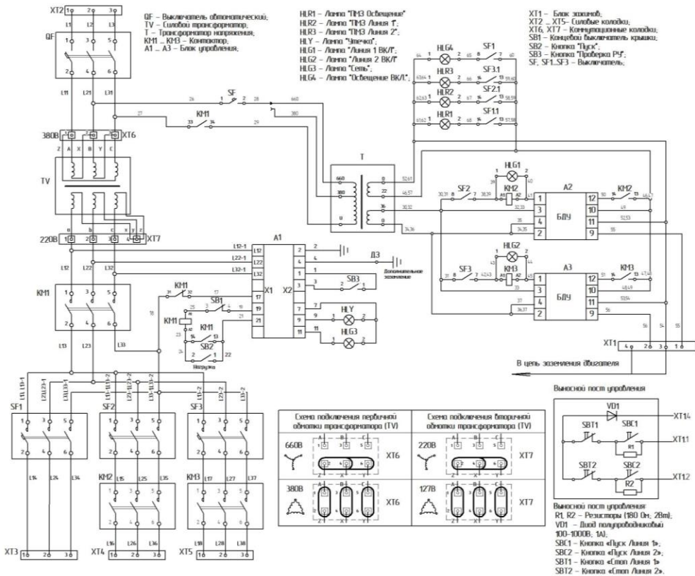
Схема электрическая АПР 660-380/220-127В.
